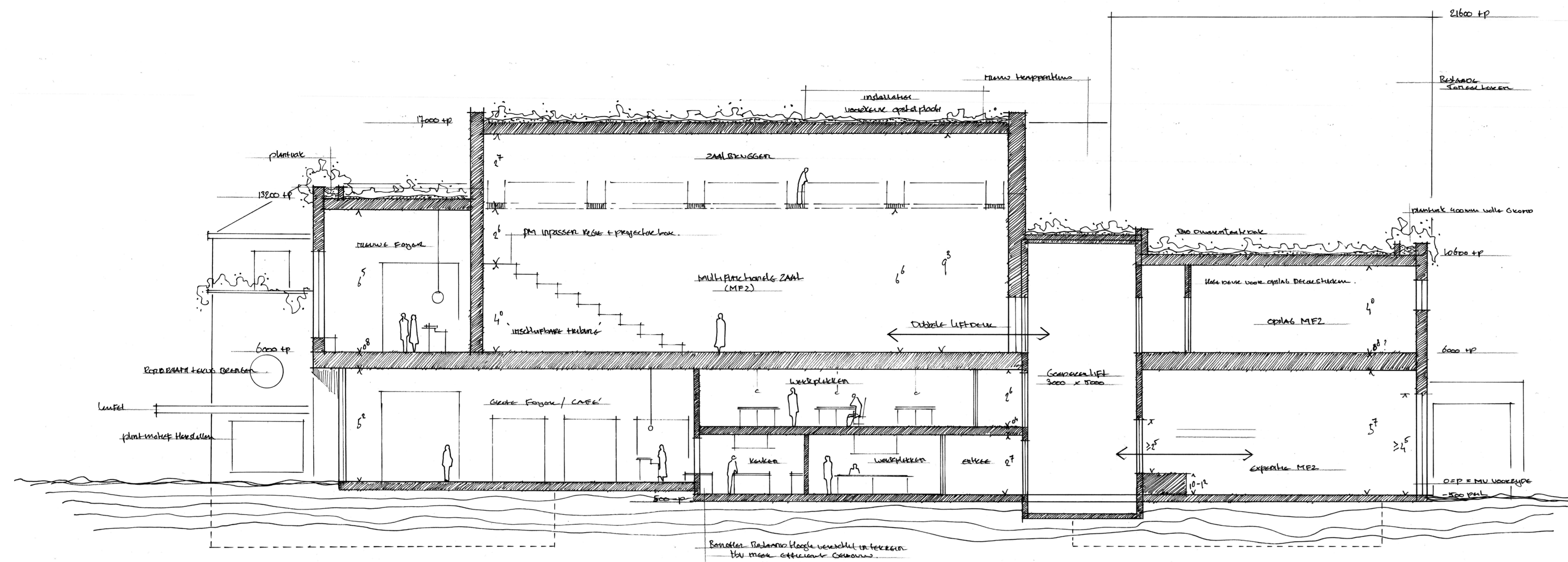
DWARSDOORSNEDE
